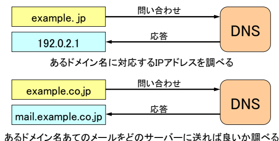
図 1: DNS の使用例
